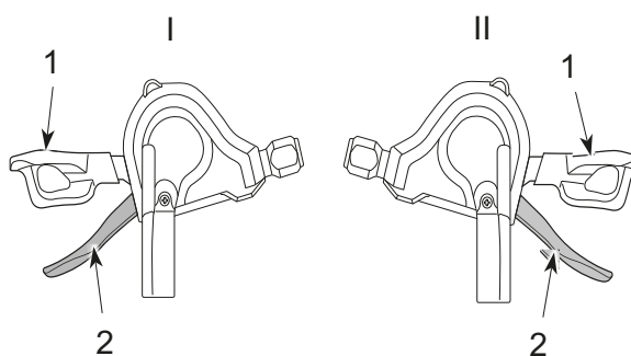
Illustration 84 : Manette de vitesse inférieure (1) et manette de vitesse supérieure (2) du changement de vitesse gauche (I) et droit (II)
