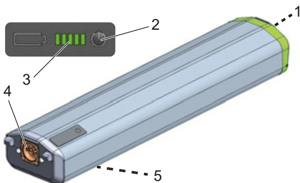
Illustration 15 : Détail de la batterie SuperCore
