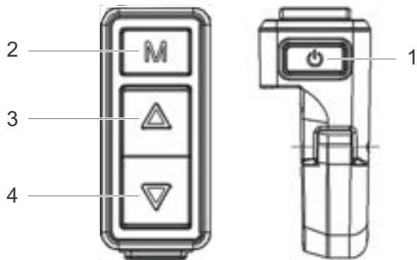
Illustration 17 : Aperçu de l'élément de commande
