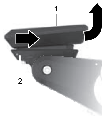
Abbildung 110: Bordcomputer abnehmen.
