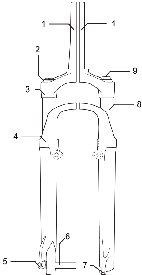
Abbildung 13: Beispiel Stahlfedergabel Suntour
