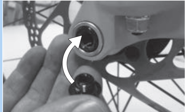
Abbildung 55: Sicherungsschraube einsetzen
