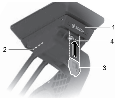
Abbildung 109: Lage Steuersatzschraube
