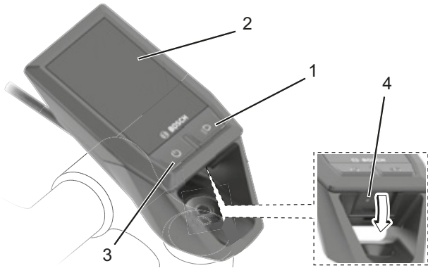
Figura 122: Vista general de la estructura y los elementos de mando del ordenador de a bordo
