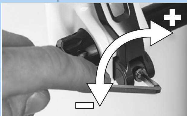
Figura 161: Ajuste de la fuerza de tensado del cierre rápido
