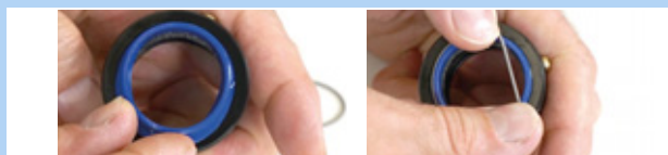
Figura 212: Inserción y fijación del rascador
