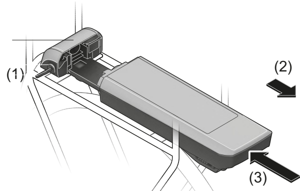
Figura 47: Extracción (2) e inserción (3) de la batería del portaequipajes
