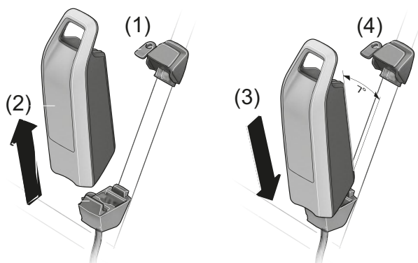
Figura 136: Extracción e inserción de la batería en el cuadro
