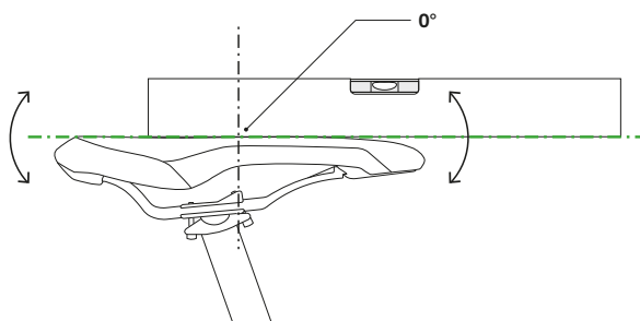
Figura 92: Inclinación del sillín horizontal con 0° de inclinación en el centro del sillín
