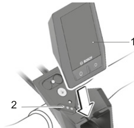
Figura 123: Colocación del ordenador de a bordo (1)
