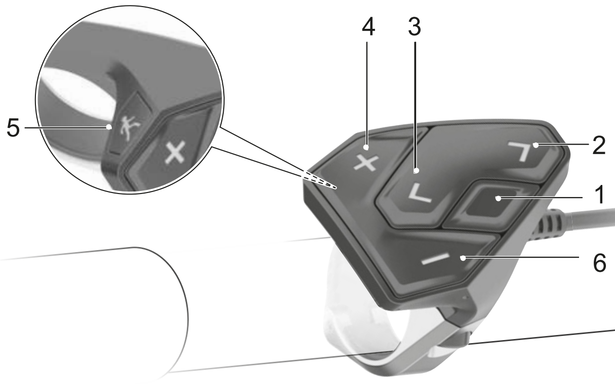
Figura 43: Vista general de la unidad de mando BOSCH
