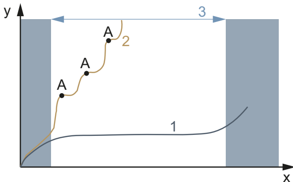
Figura 146: Diagrama de desgaste, vida útil (x) con respecto a desgaste de materiales (y)
