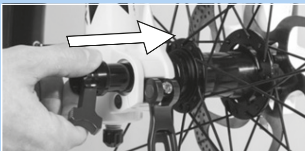
Figura 71: Inserción del eje transversal en la dirección de la flecha
