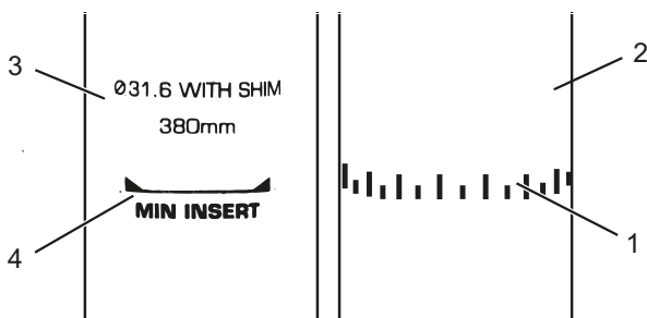
Figura 89: Vista detallada de las tijas de sillín, ejemplos de las marcas de la profundidad de inserción mínima
