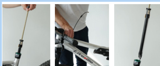
Figura 167: Extracción del cartucho
