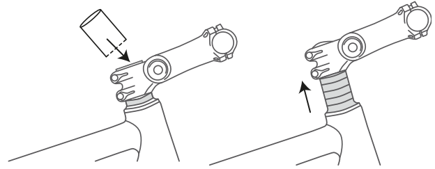
Figura 98: Aumento de la potencia Ahead mediante el montaje de anillos distanciadores (separadores)
