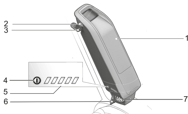
Figura 36: Detalle de la batería en el cuadro
