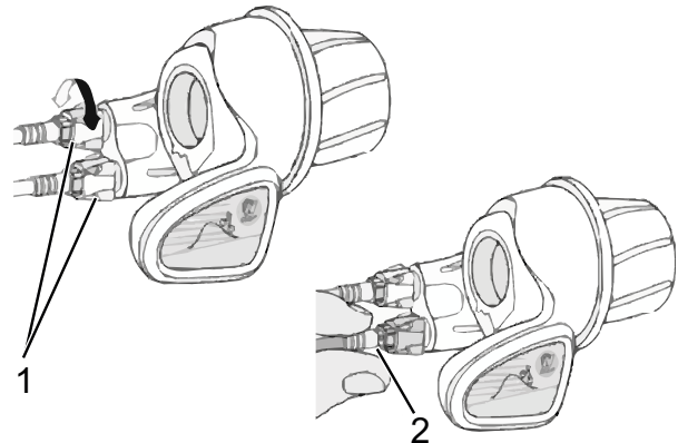
Figura 159: Puño giratorio con casquillos de ajuste (1) y holgura del cambio de marchas (2)
