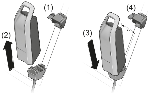
Figura 46: Extracción e inserción de la batería en el cuadro
