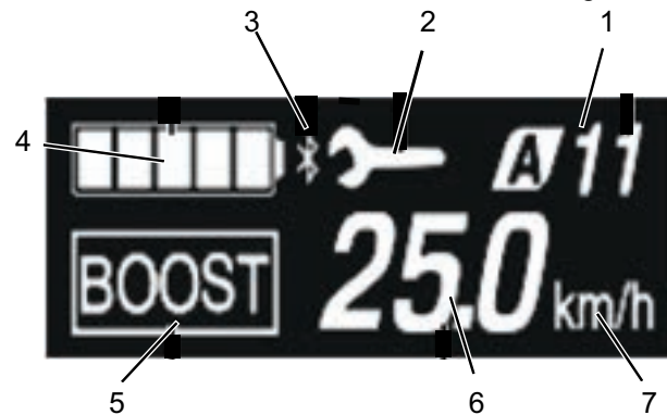
Abbildung 20: Übersicht Bildschirmanzeigen
